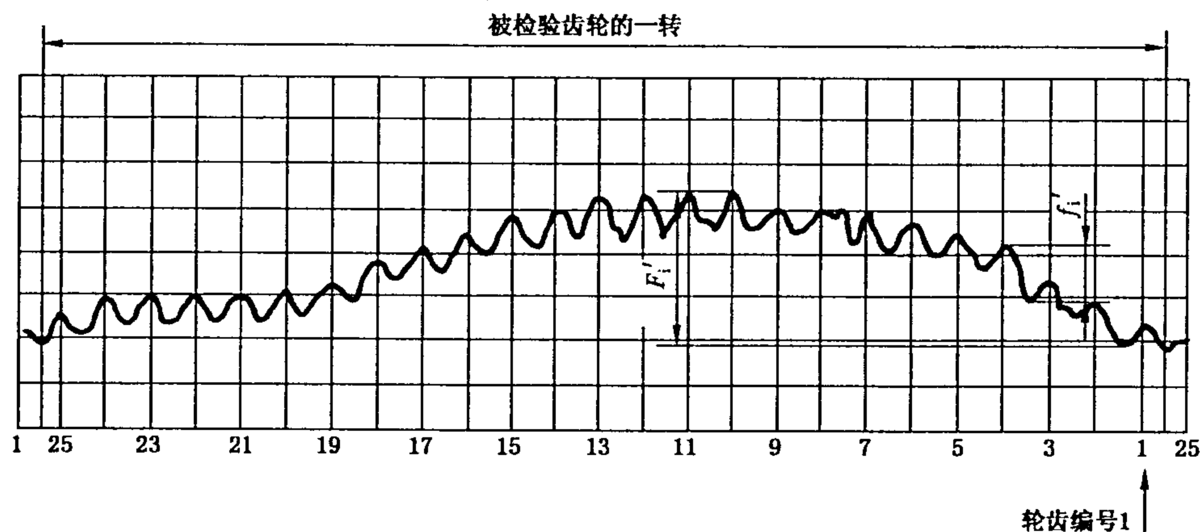
图 4 切向综合偏差
