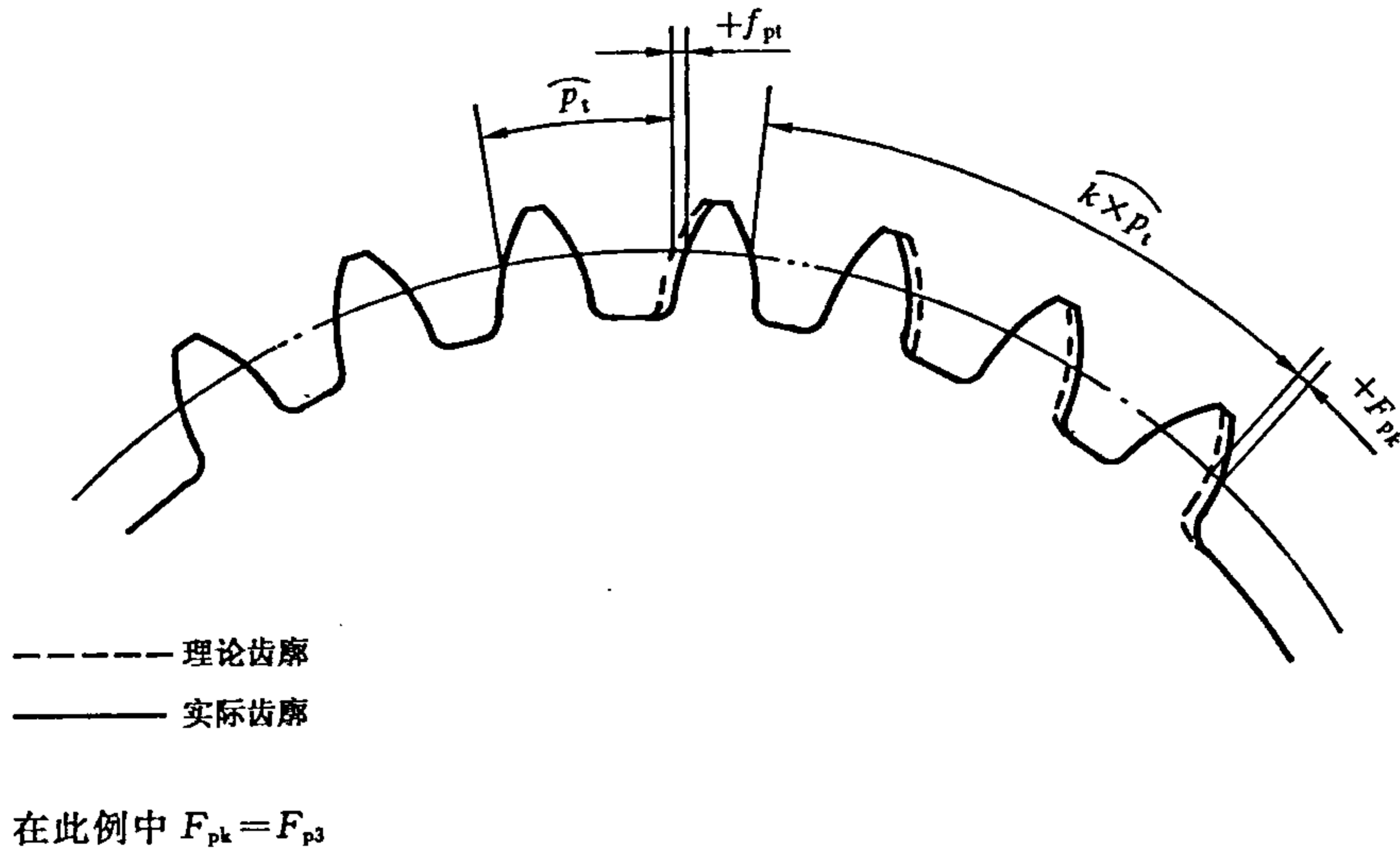
图 1 齿距偏差与齿距累积偏差
