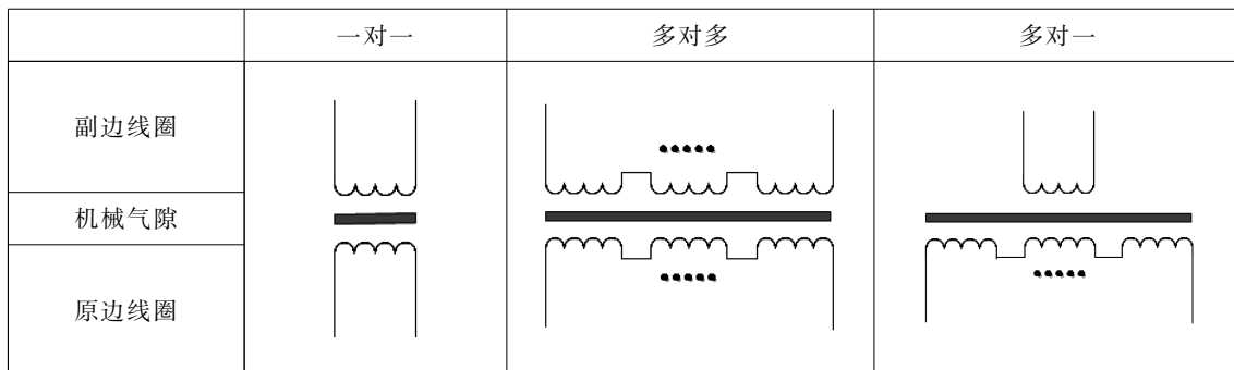
图 1 磁极结构
